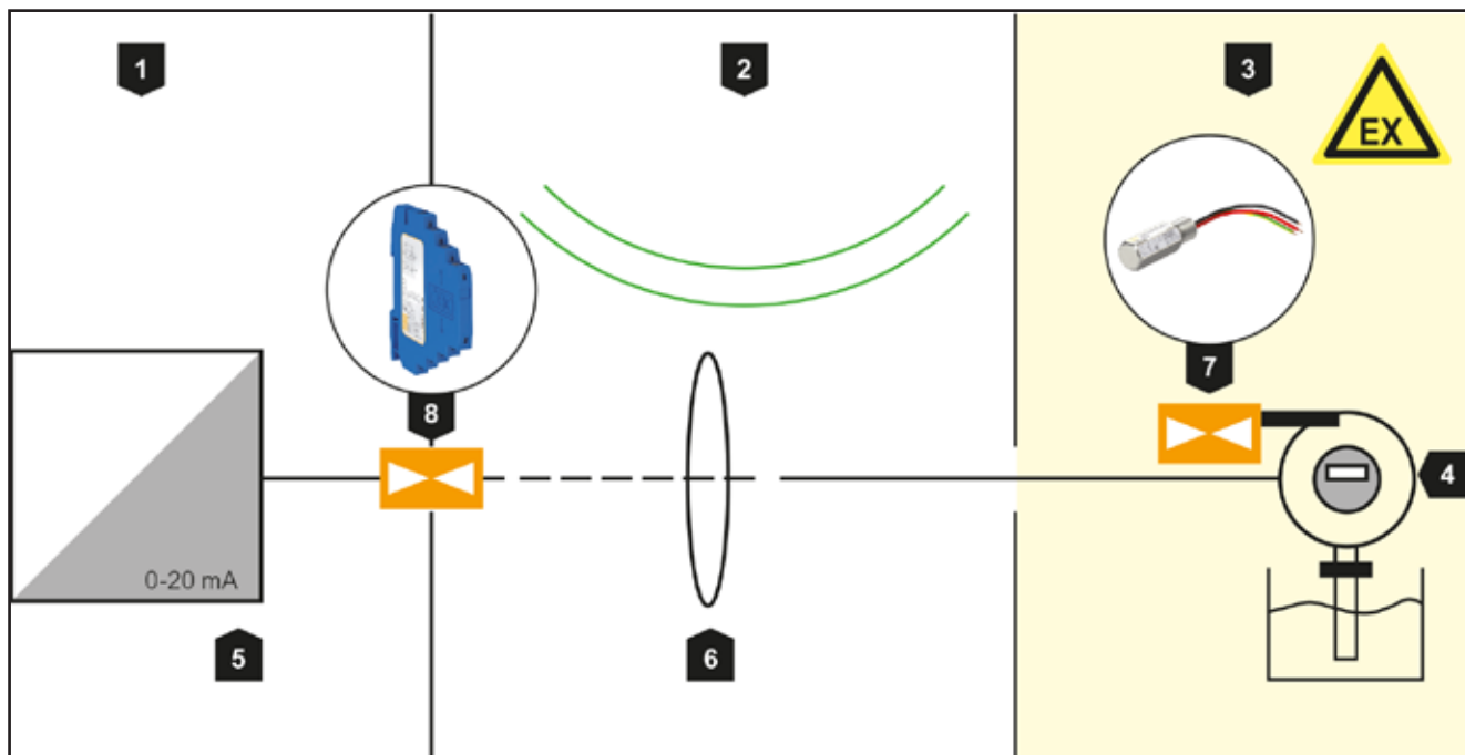
Abb. 5: Anschlussschema MDP-EX und FDB im Ex-Bereich
