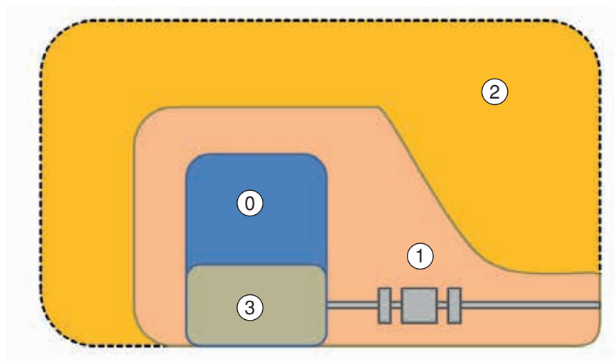
Abb. 1: Beispiel der Zoneneinteilung für Gas-Ex-Bereiche nach IEC 60079-10-1
