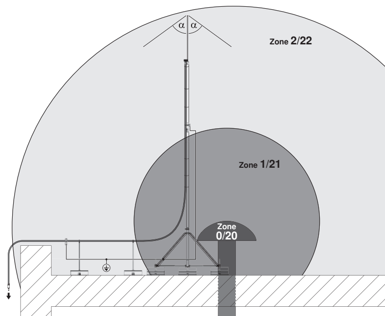
Abb. 8: Beispiel für die Installation des isCon®Pro+ -Systems in den Ex-Zonen eines explosionsgefährdeten Bereichs
