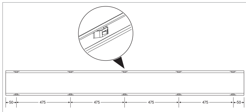
Abb. 31: Anzahl und Abstände der Rastsicken im Kanaldeckel.
