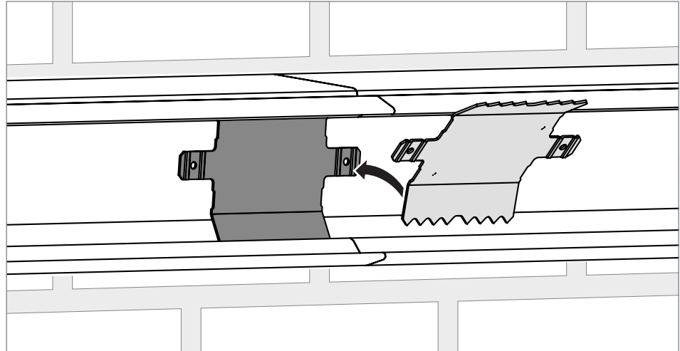
Abb. 30: Verbinder PLM 0404 montieren
