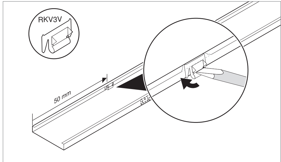
Abb. 34: Einsetzen einer Rastklemme am abgelängten Kanaldeckel.
