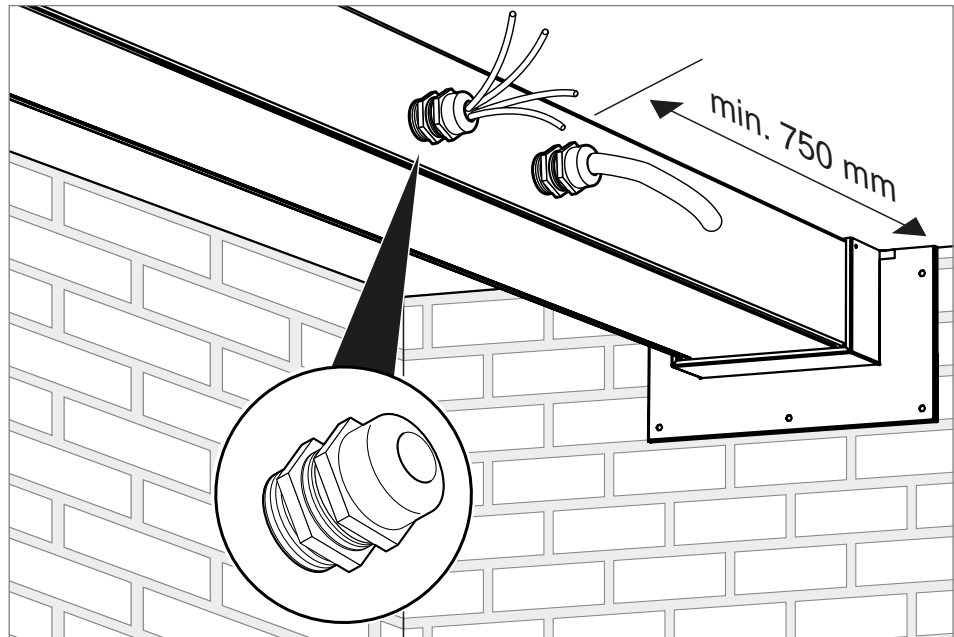
Abb. 37: Einzelkabelausgang herstellen
