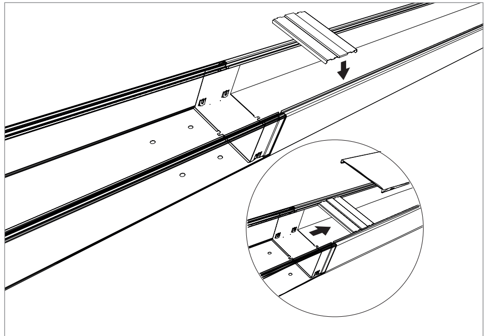
Abb. 32: Deckelunterstützung versetzt zu Kanalstoßstelle einsetzen.
