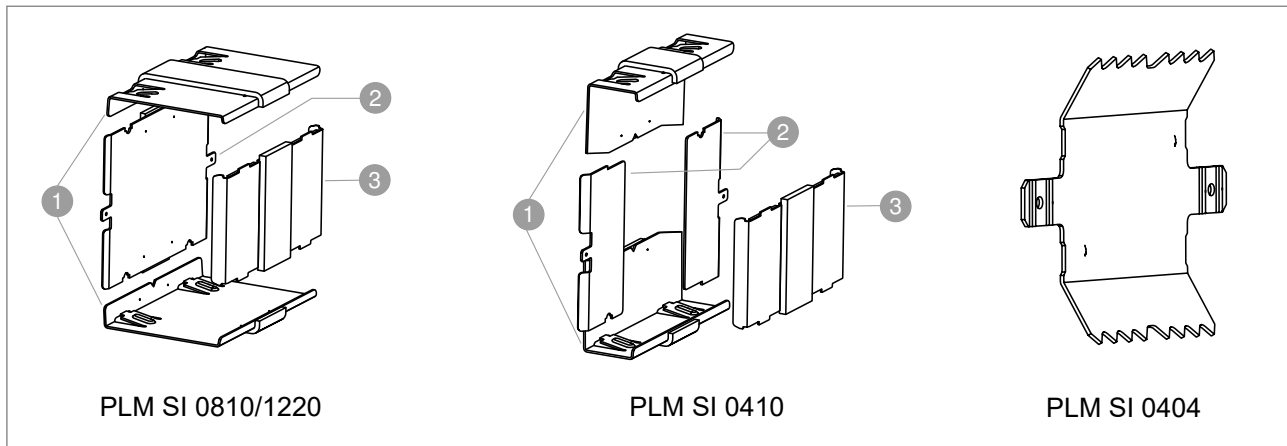
Abb. 25: Stoßstellenverbinder PLM SI...
