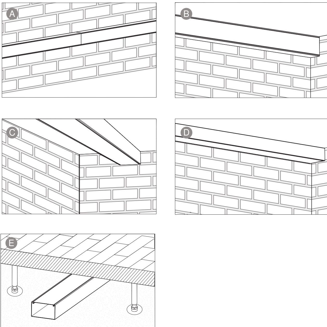
Abb. 3: Übersicht Direktmontage
