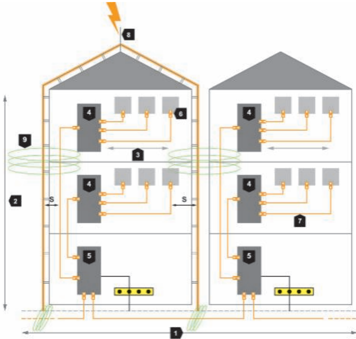
Prinzipielle Blitzstrom- und Überspannungsaufteilung in einem Gebäude mit strukturierter Verkabelung
