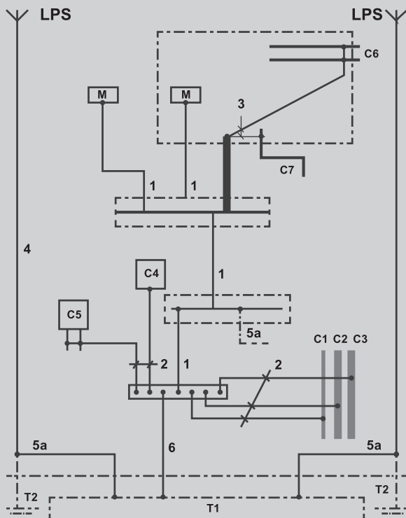
Potentialausgleich einer baulichen Anlage
