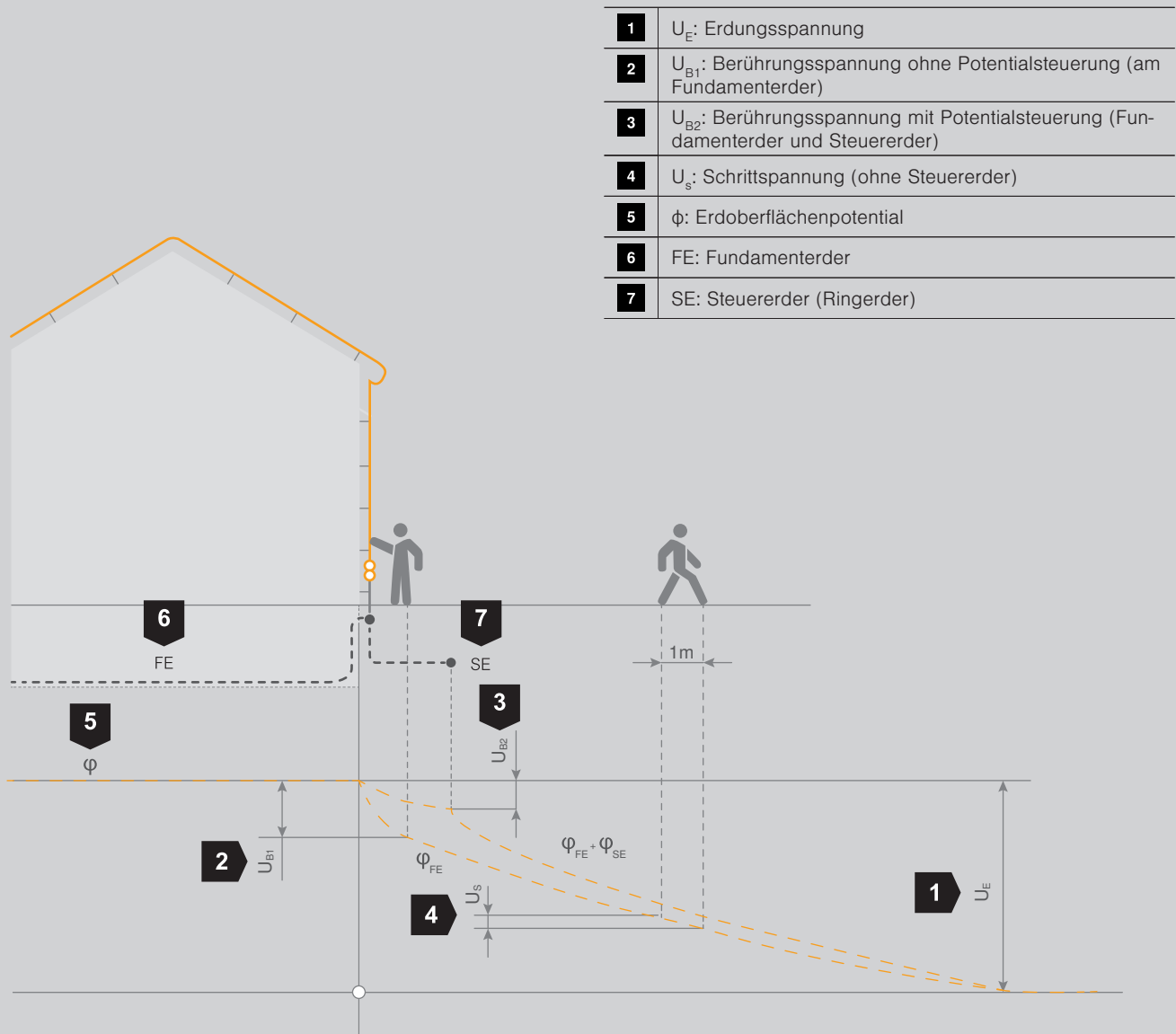
Erdoberflächenpotential und Spannungen beim stromdurchflossenen Fundamenterder FE und Steuererder SE
