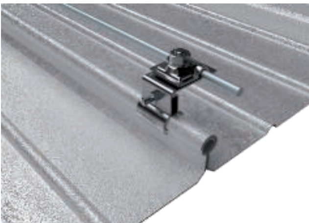
Blitzstromtragfähige Kalzip®-Klemme von OBO
