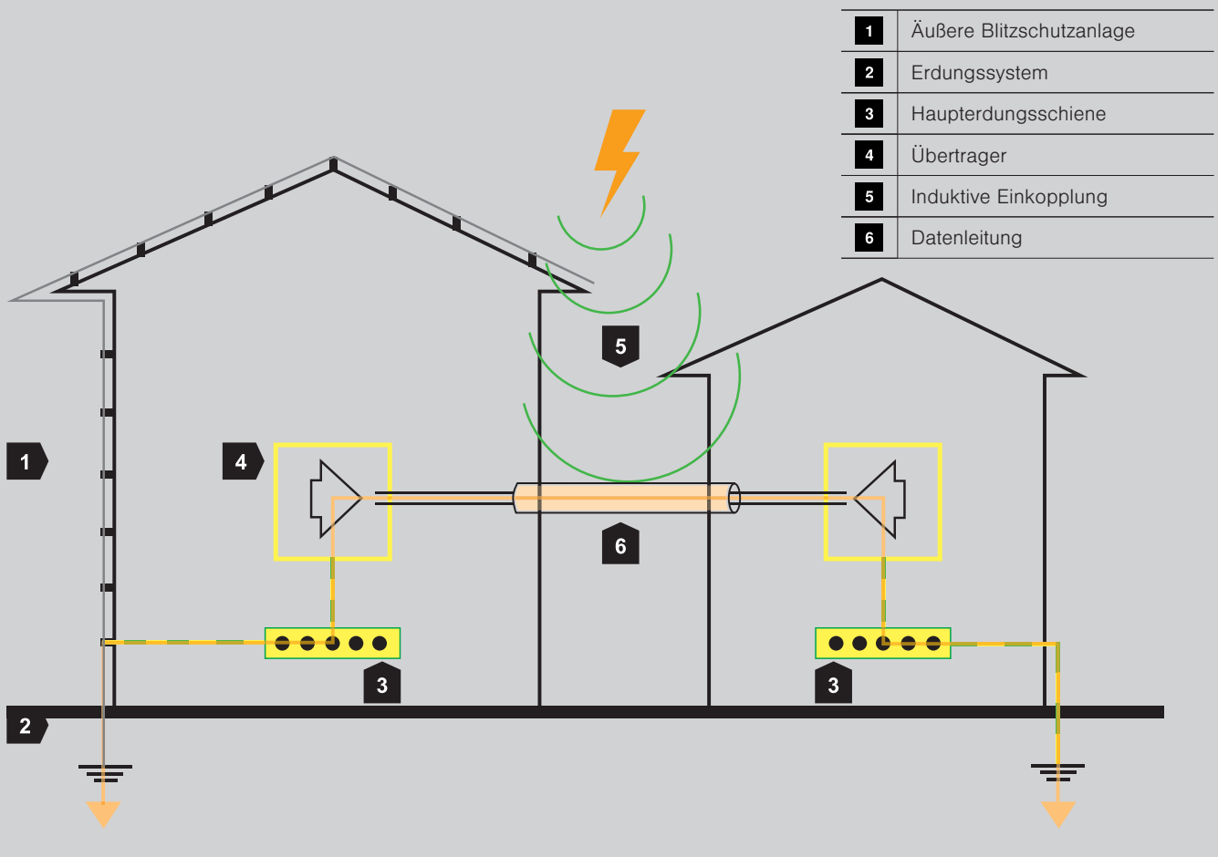
Induktive Einkopplung bei einem Direkteinschlag
