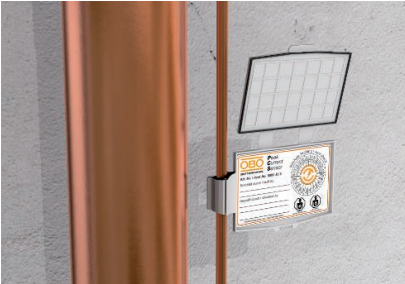
PCS-Sensor an einer Ableitung
