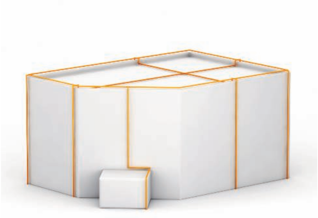
Ableitungseinrichtung nach VDE 0185-305-3 (IEC 62305-3)
