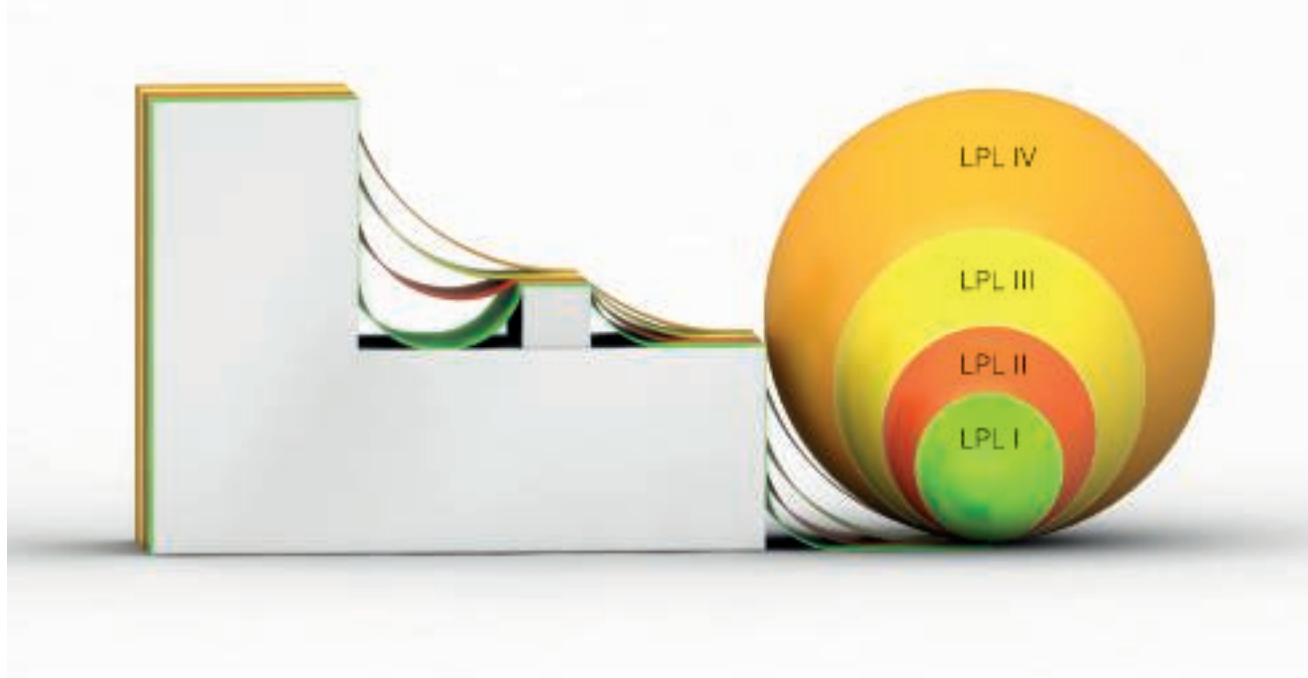
Blitzkugelradius in Abhängigkeit von der Blitzschutzklasse
