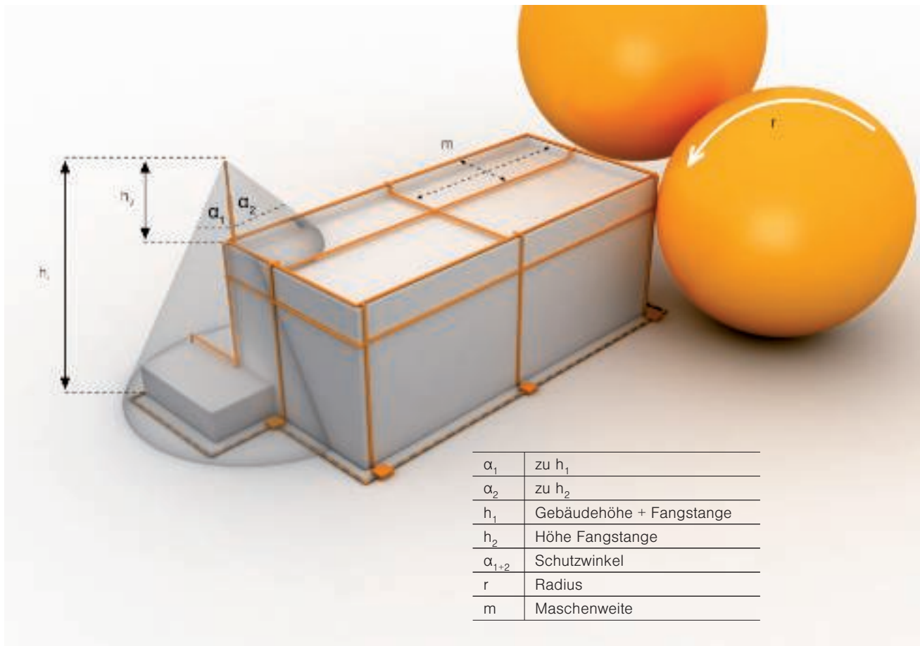
Planung mit dem Schutzwinkel-, Maschen- und Blitzkugelverfahren
