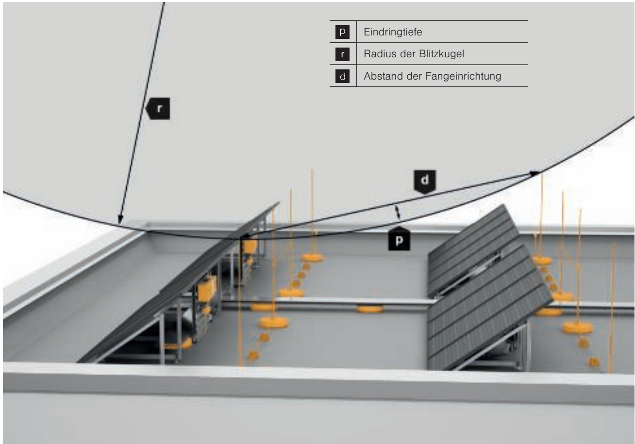
Eindringtiefe (p) der Blitzkugel zwischen den Fangstangen
