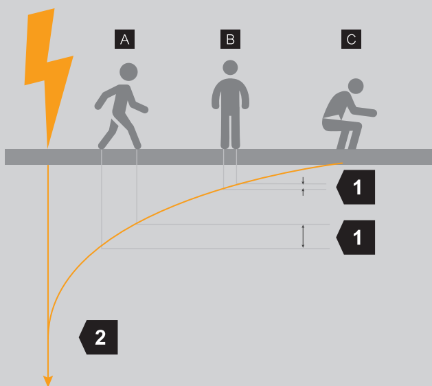
Schrittspannung und Potentialtrichter beim Blitzeinschlag
