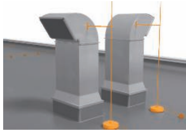
Fangstange mit verstellbarer Isoliertraverse
