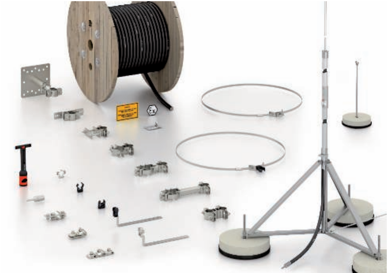
Komponenten des isCon®-Systems
