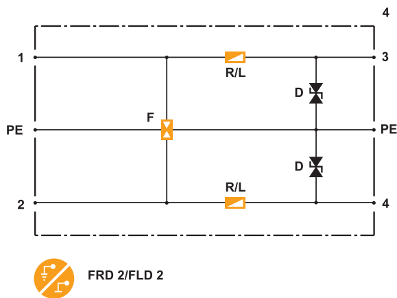
Schaltbild der Blitzbarriere FRD2/FLD2
