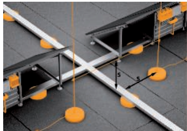
PV-Anlage im Schutzbereich der Fangeinrichtung im Trennungsabstand (s)
