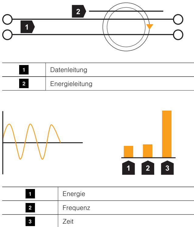
Induktive Einkopplung durch eine parallel verlegte Energieleitung
