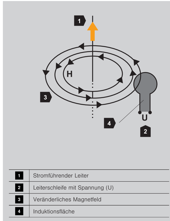
Induktion in einer Leiterschleife
