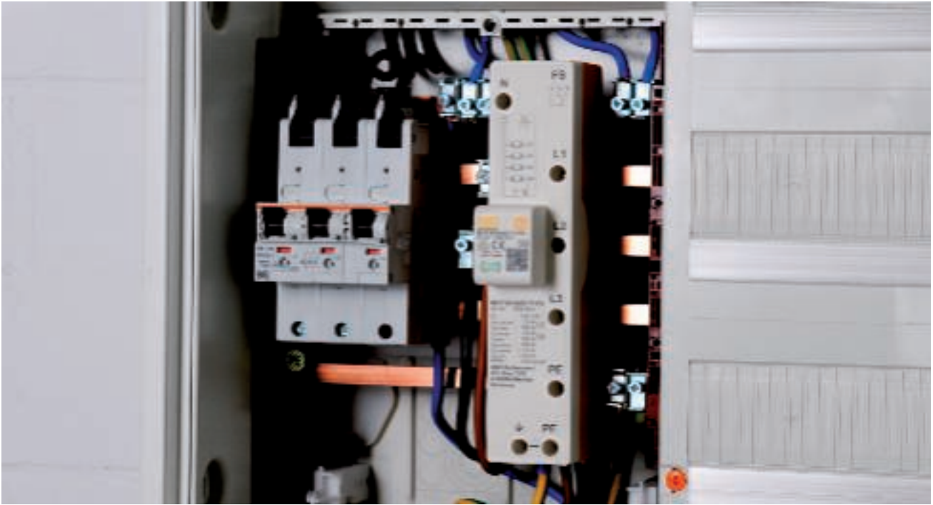
Typ 1+2 Kombiableiter MCF...NAR auf der 40-mm-Sammelschiene im netzseitigen Anschlussraum
