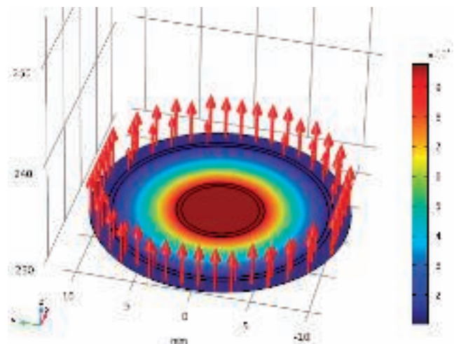
Stromdichtevektoren in der resistiven Feldsteuerung und Potentialdichte einer isolierten Ableitung zum Zeitpunkt t = 1,2 \mu\text{s} der angelegten Impulsspannung 1,2/50 20 cm unterhalb der geerdeten Befestigungsklemme. Am Innenleiter liegt ein Potential von 1000 kV.
