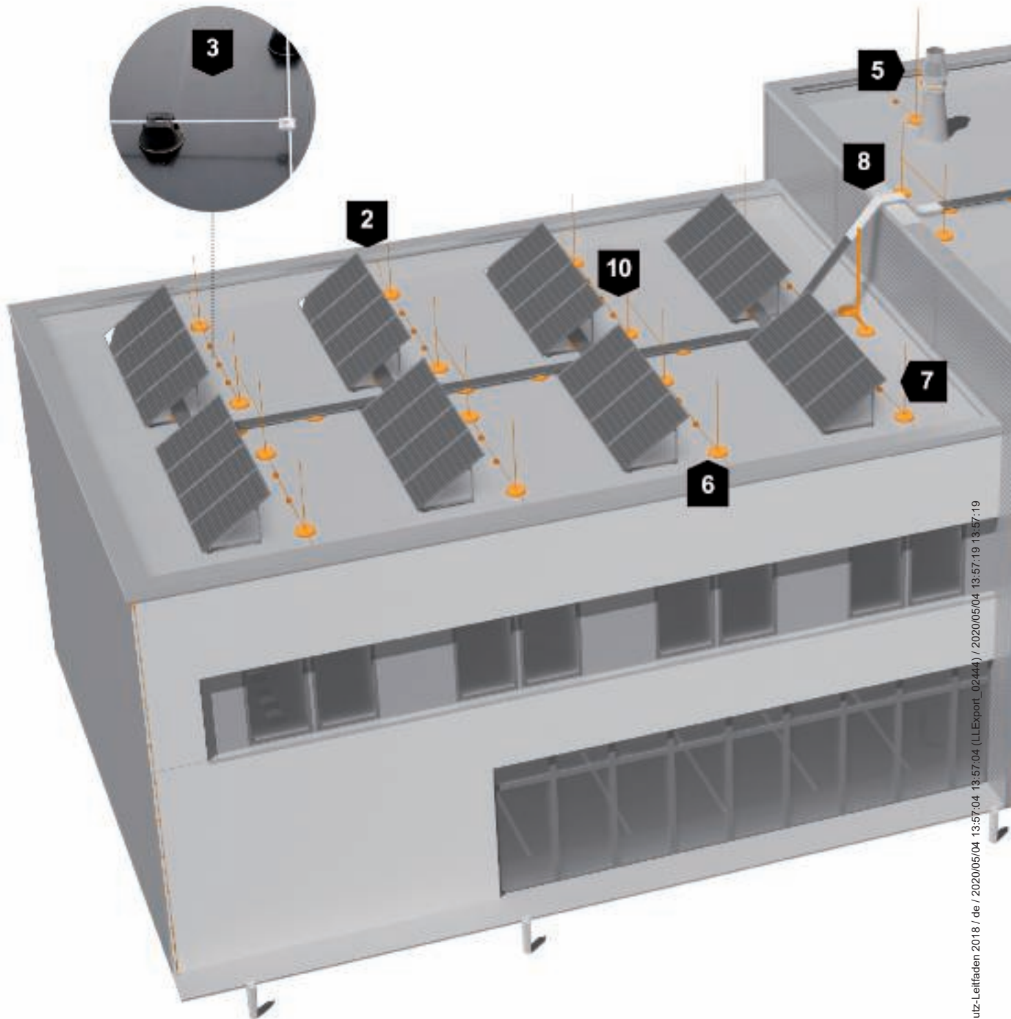
Gebäude mit Flachdach und Blitzschutzsystem
