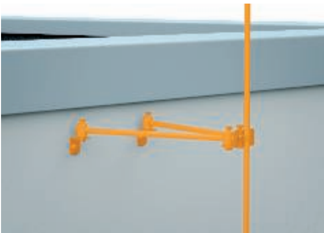
Beispiel: Fangsystem mit Iso-Combi-Set für V-Befestigung
