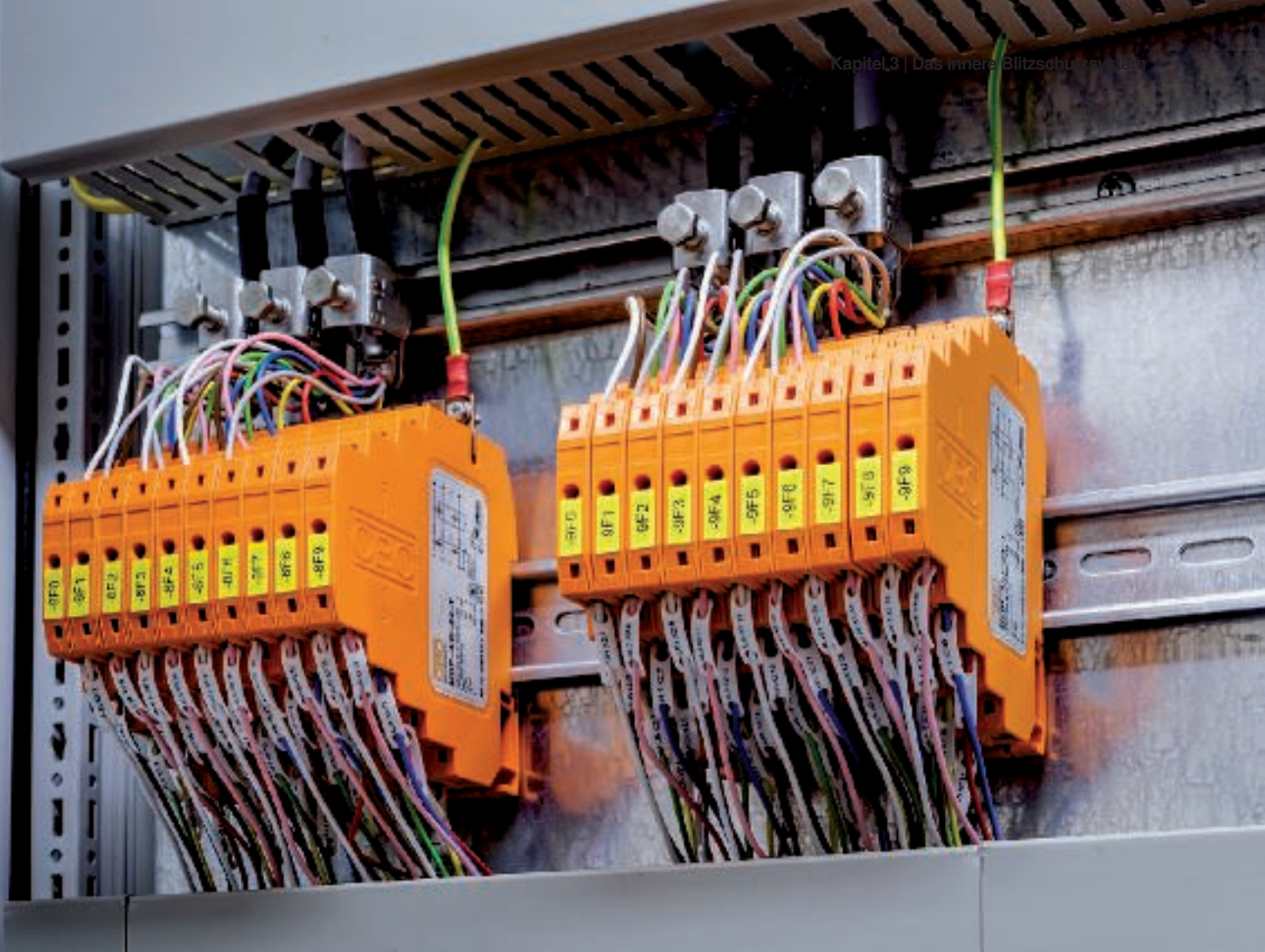
Installationen der MDP-Blitzbarriere im Schaltschrank
