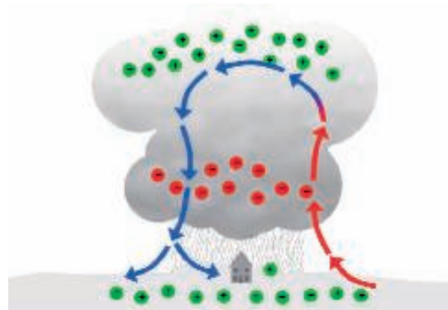
Blitzentstehung durch Ladungstrennung
