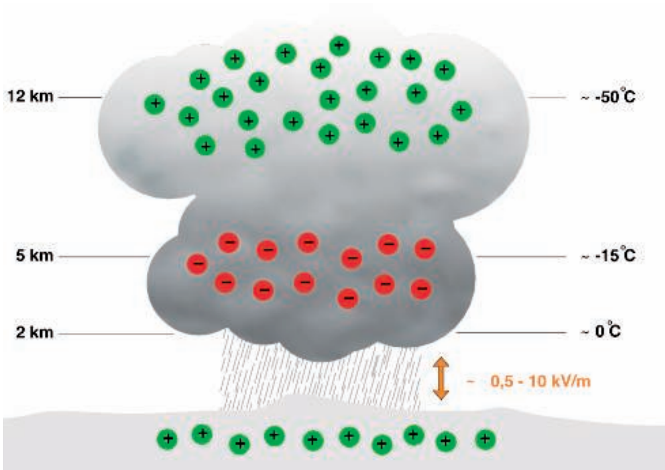
Ladungsverteilung in einer Wolke
