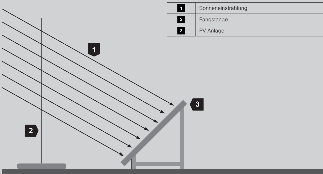
Beschattung eines PV-Moduls durch eine Fangstange
