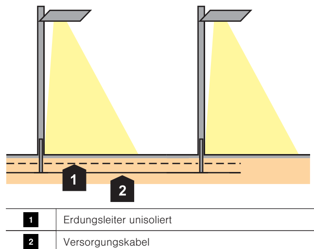
Leitungsführung
