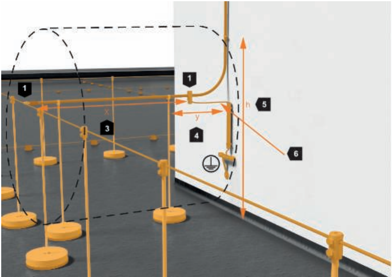
Beispiel: isCon®-Ableitung an getrennter Ringleitung
