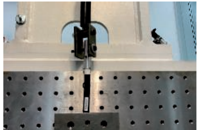
Prüfaufbau der statisch mechanischen Belastung
