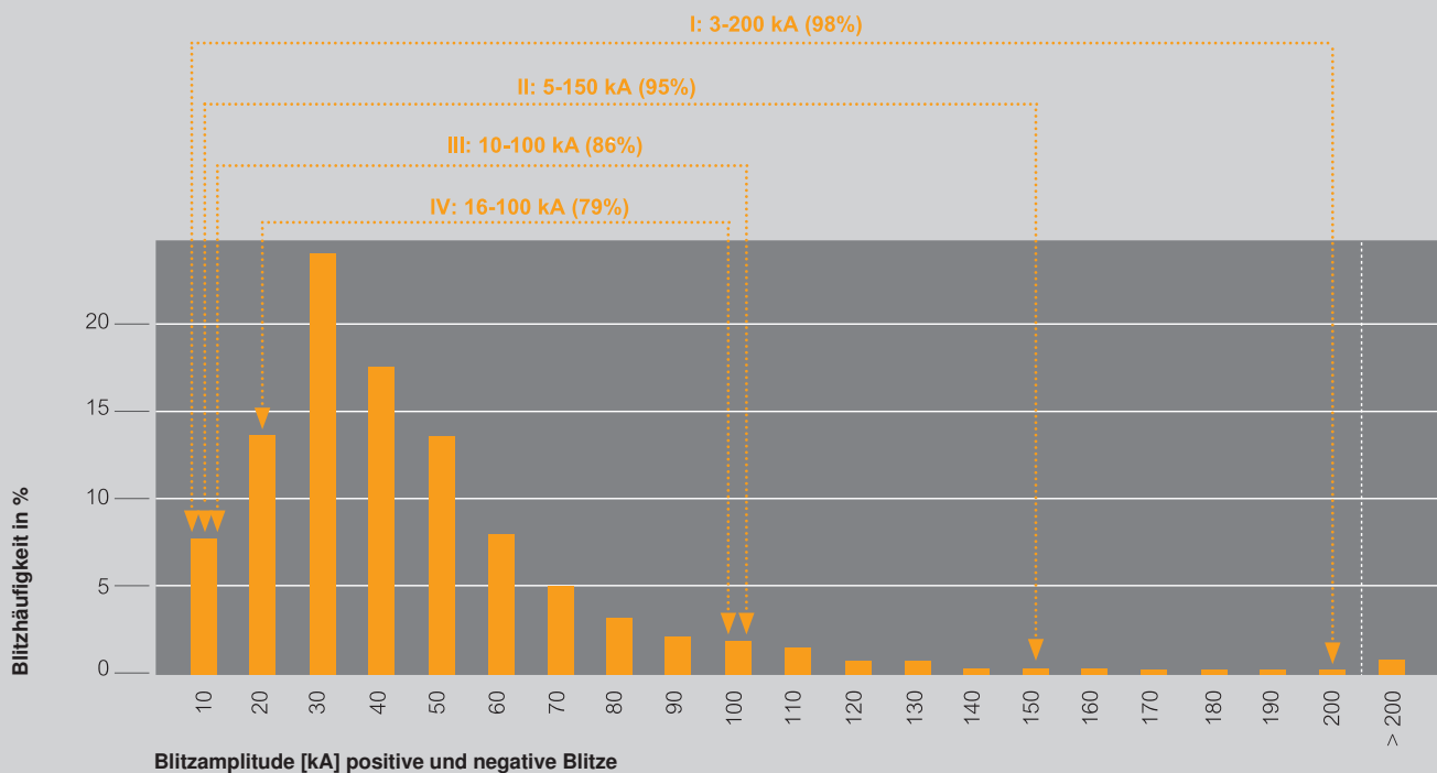
Blitzstromparameter entsprechend des Gefährdungspegels LPL nach VDE 0185-305-1
