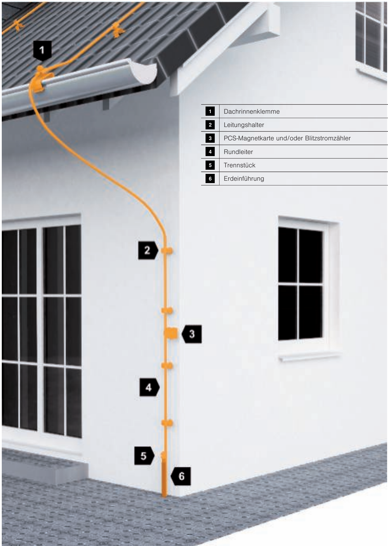
Installationsprinzip Ableitungseinrichtung
