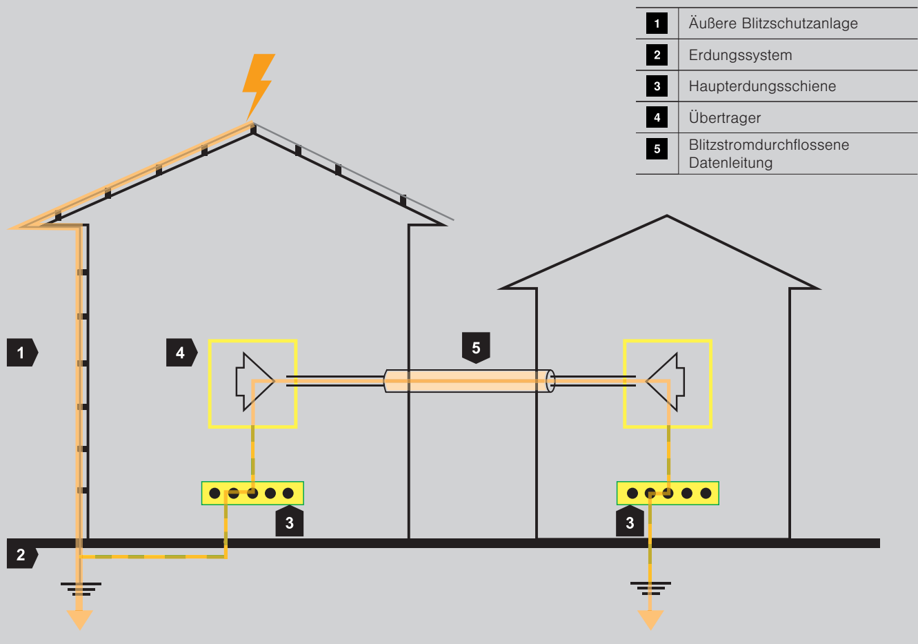
Galvanische Einkopplung in eine Datenleitung über die äußere Blitzschutzanlage
