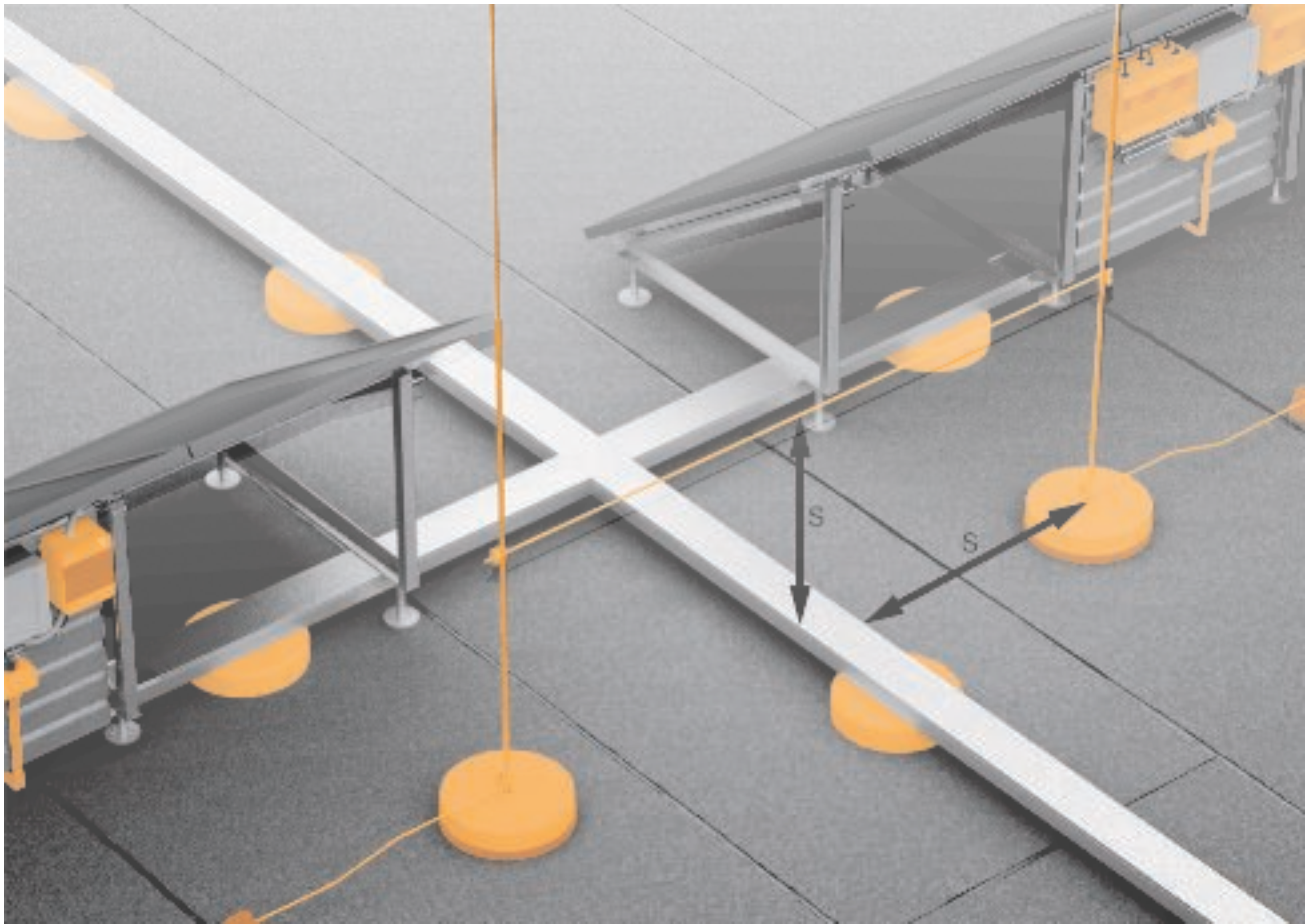
Isolierter Blitzschutz mit eingehaltem Trennungsabstand (s)
