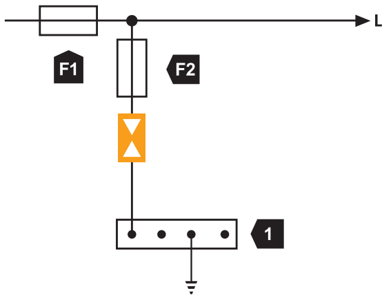
Vorsicherung an Überspannungsschutzgeräten
