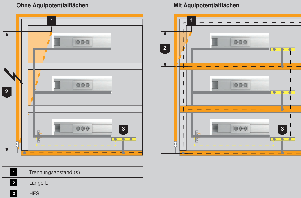
Trennungsabstand bei hohen Gebäuden ohne und mit Äquipotentialfläche als Bezugsebene
