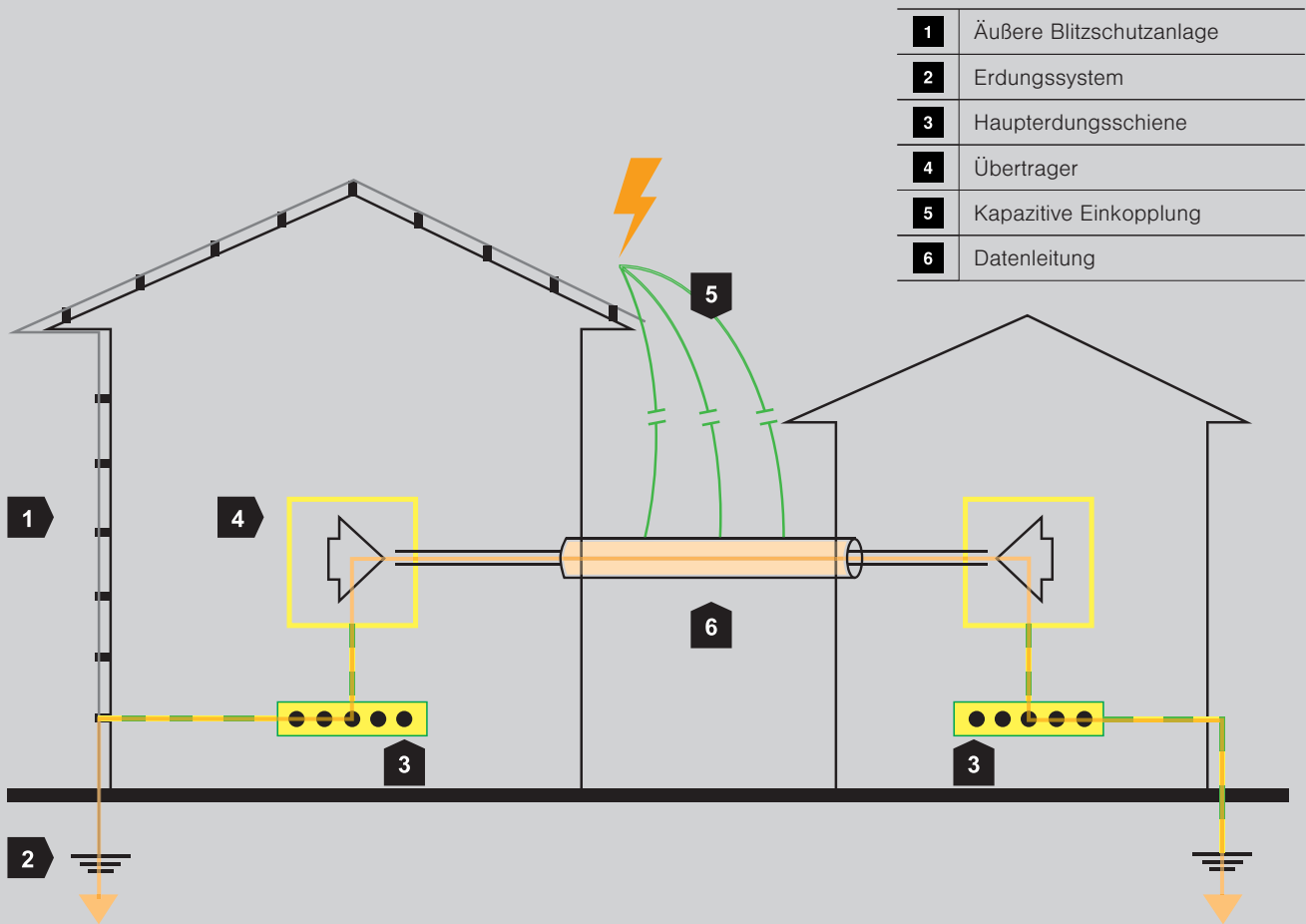
Kapazitive Einkopplung bei Direkteinschlag
