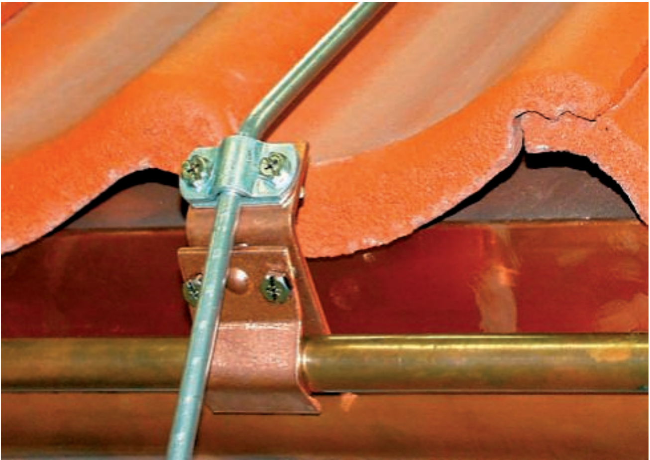
Zweimetall-Dachrinnenklemme (Aluminiumrundleiter und Kupferdachrinne)
