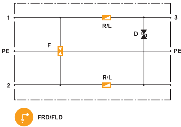
Schaltbild der Blitzbarriere FRD/FLD
