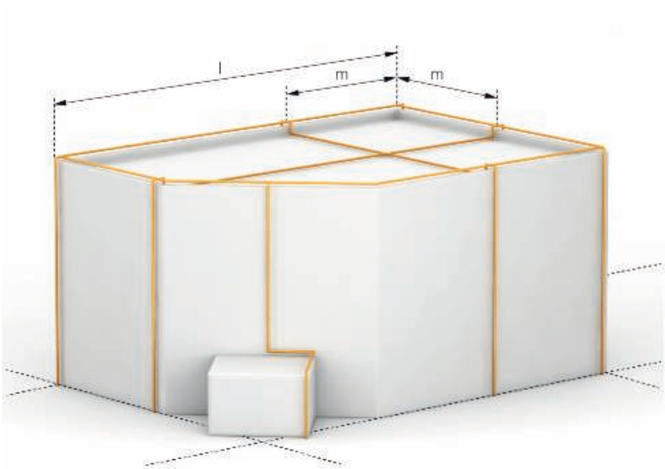
Maschensystem auf einem Flachdach
