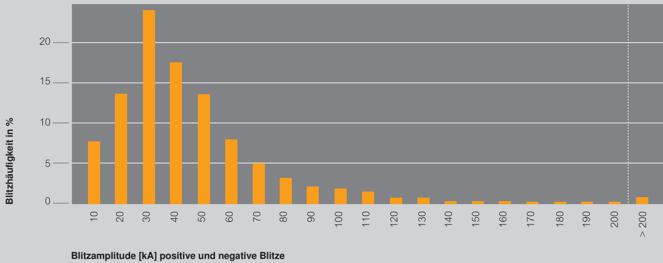
Teilung der Blitzhäufigkeit zur Blitzamplitude
