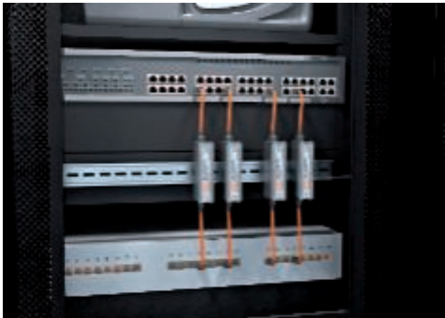
Schutzvorschlag am Switch mit Patchfeld. Die Überspannungsschutzgeräte sind über die Hutschiene geerdet.
