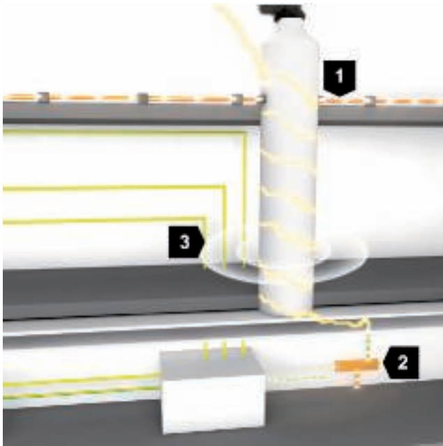
Getrenntes System mit GFK-Haltern
