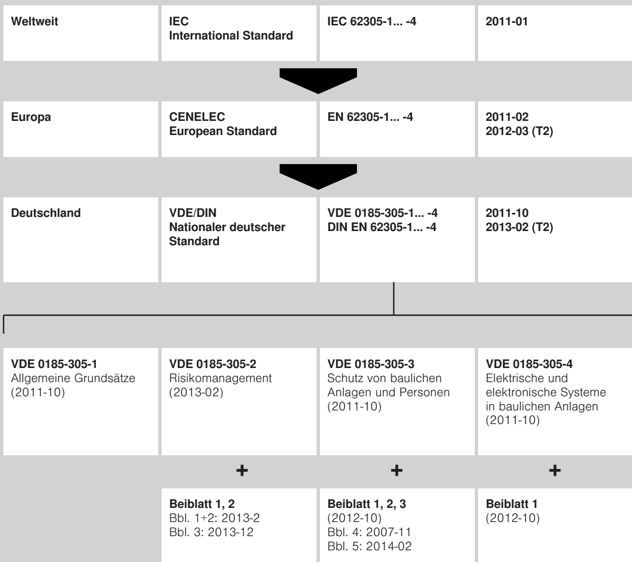
Hierarchie der Blitzschutznormung (international/europäisch/national) und Stand der deutschen Blitzschutznormung: Normung und Vorschriften
