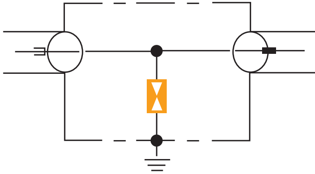
Koaxiales Überspannungsschutzgerät mit Gasableiter
