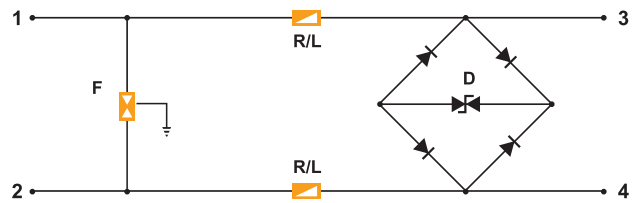
Grundschutzschaltung im Messkreis
