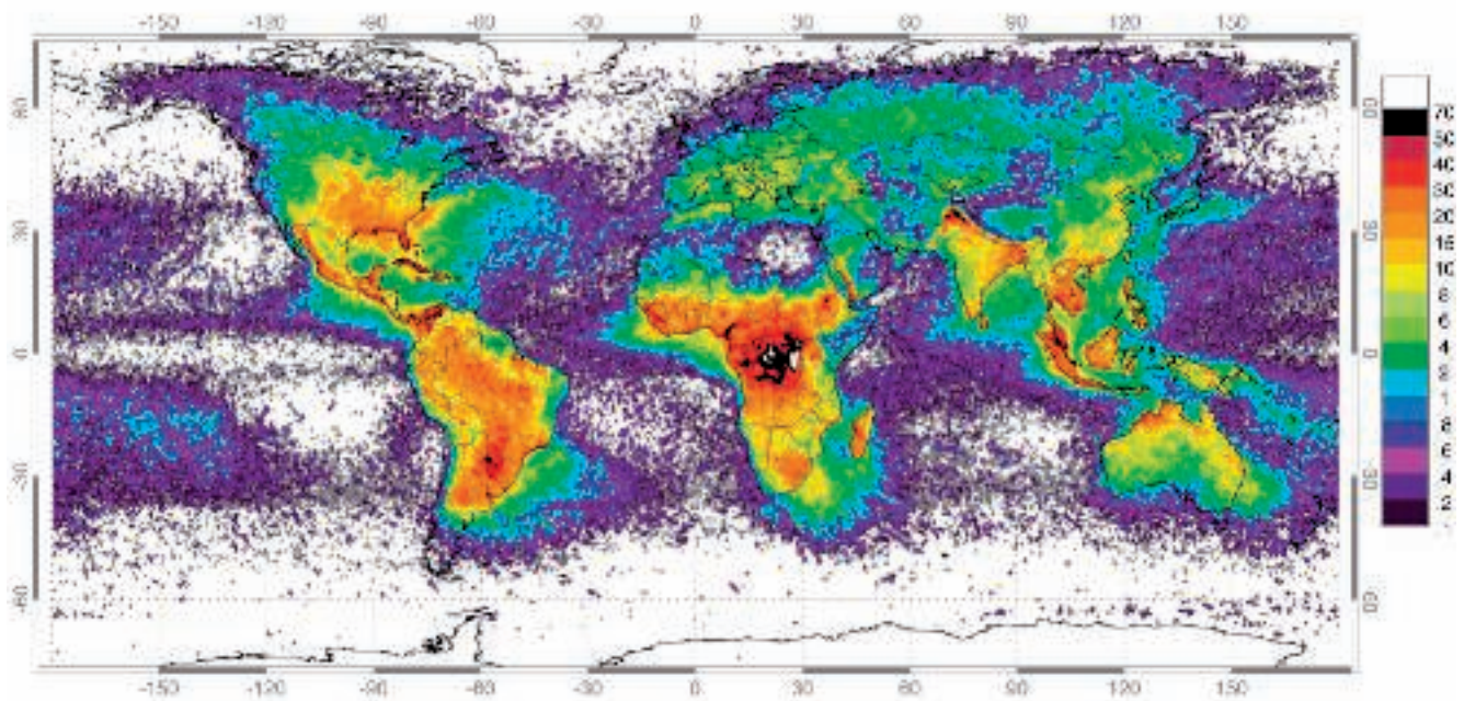
Blitzdichte als jährliche Anzahl von Blitzeinschlägen pro km 2 im Zeitraum von 1995 bis 2003 ( www.nasa.gov )
