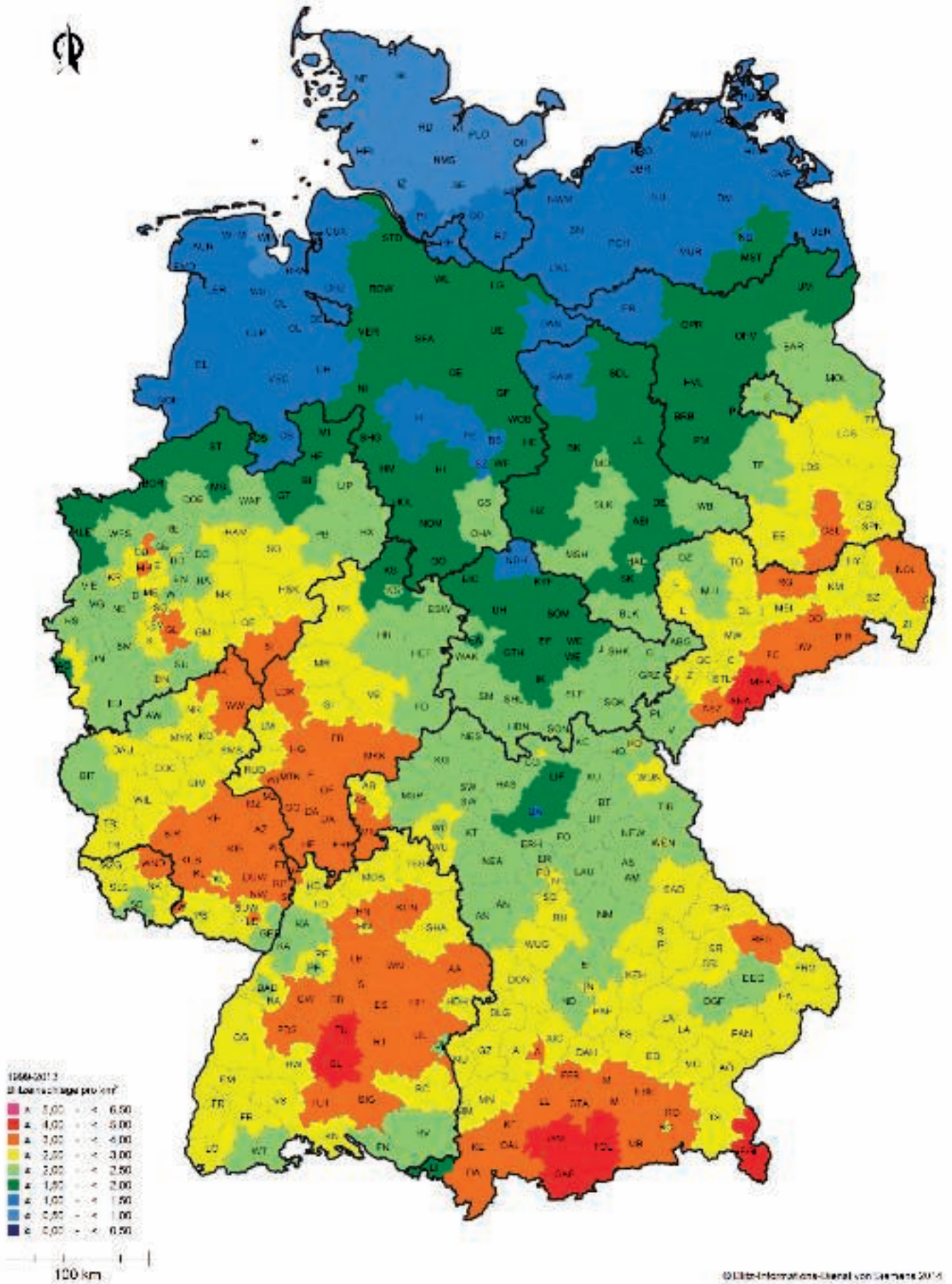
Blitzhäufigkeit in Deutschland. Quelle: www.siemens.com
