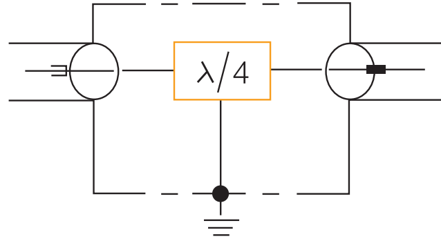
Koaxiales Überspannungsschutzgerät mit Lambda/4 Technologie
