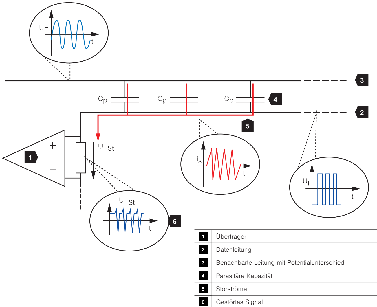
Auswirkung einer kapazitiven Einkopplung auf einen Übertrager
