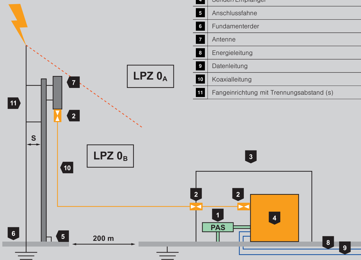
Isolierter Blitzschutz an Antennenanlage und unterschiedlichen Erdungssystemen
