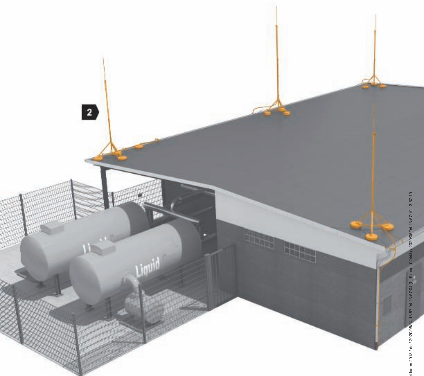
Installationsprinzip isCon® in explosionsgefährdeten Bereichen
